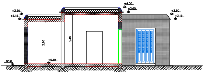
ΤΟΜΗ Β-Β'
