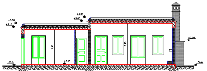
ΤΟΜΗ Α-Α'
